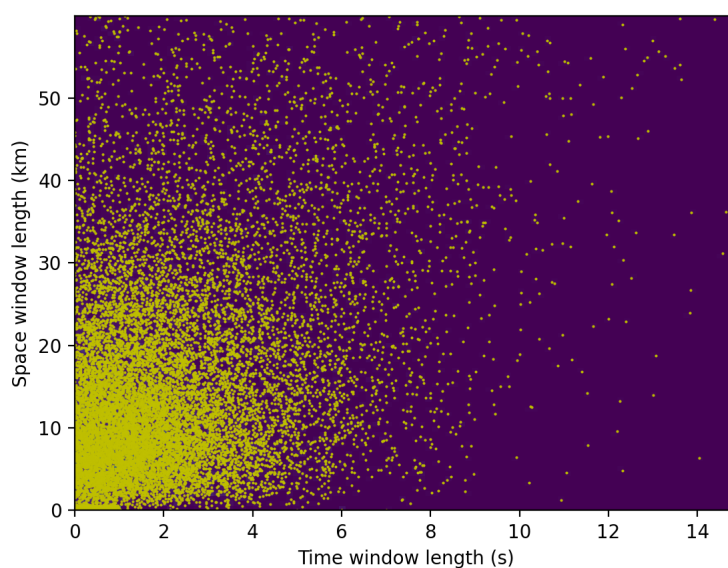
Рисунок 2. Расстояние во времени и пространстве для событий, идентифицированных как дублирующиеся, из бюллетеня ISC и каталога ЕМСА. Более 95% событий попадает в окно 15 с и 60 км, хотя основная масса событий находится в пределах ошибки 5 с и 25 км. По горизонтальной оси отложена длина временного окна в секундах, по вертикальной оси - длина пространственного окна в километрах
