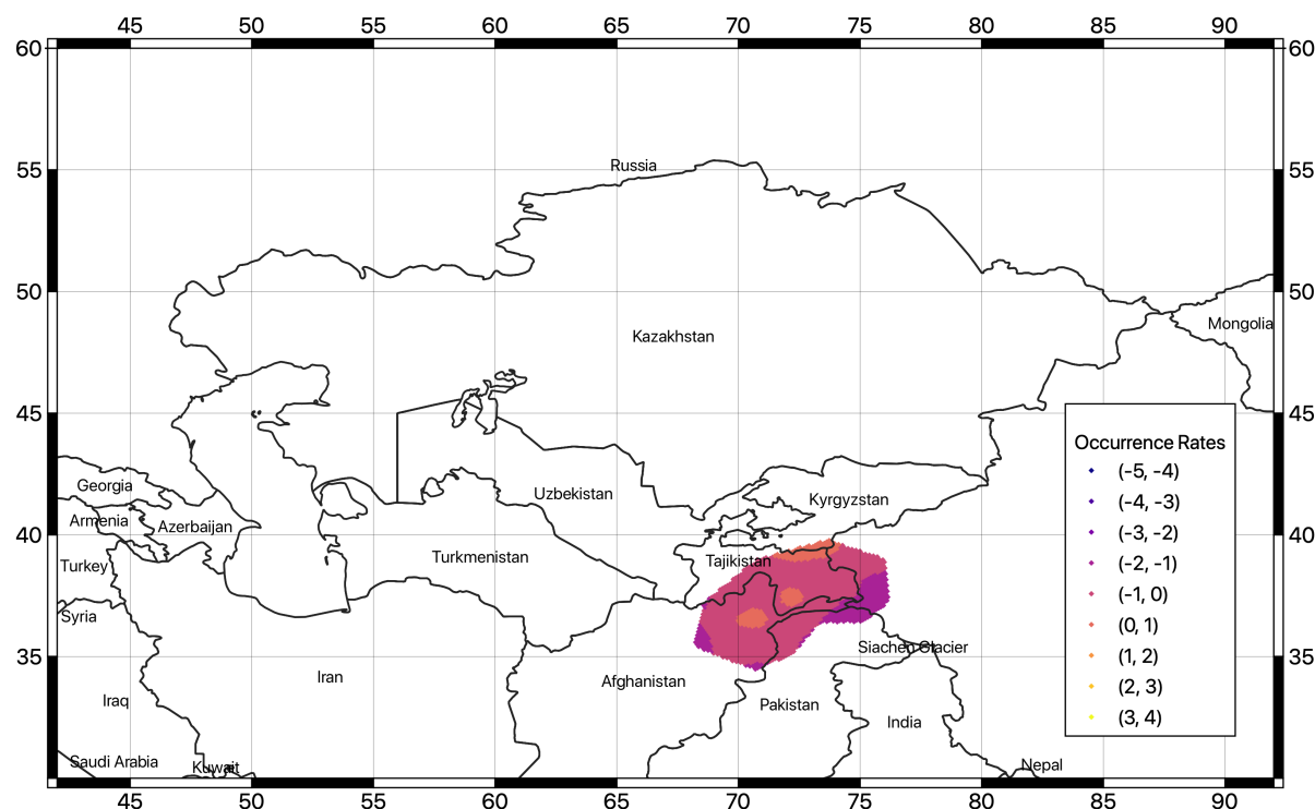
Рисунок 18. Пространственное распределение степени проявления событий в сглаженном виде для зон глубоких землетрясений. Посчитаны с учетом среднего значения весов длины шага сглаживания из Таблицы 13.
