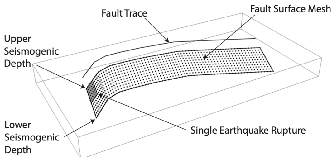
Рисунок 19. Представление источника в виде простого разлома в OpenQuake.
