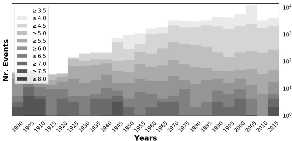
Рисунок 6. Количество событий каталога Центральной Азии, рассчитанное для пятилетних окон за период 1900-2015 гг. Штриховка соответствует ячейкам с возрастающей пороговой магнитудой (кумулятивная)
