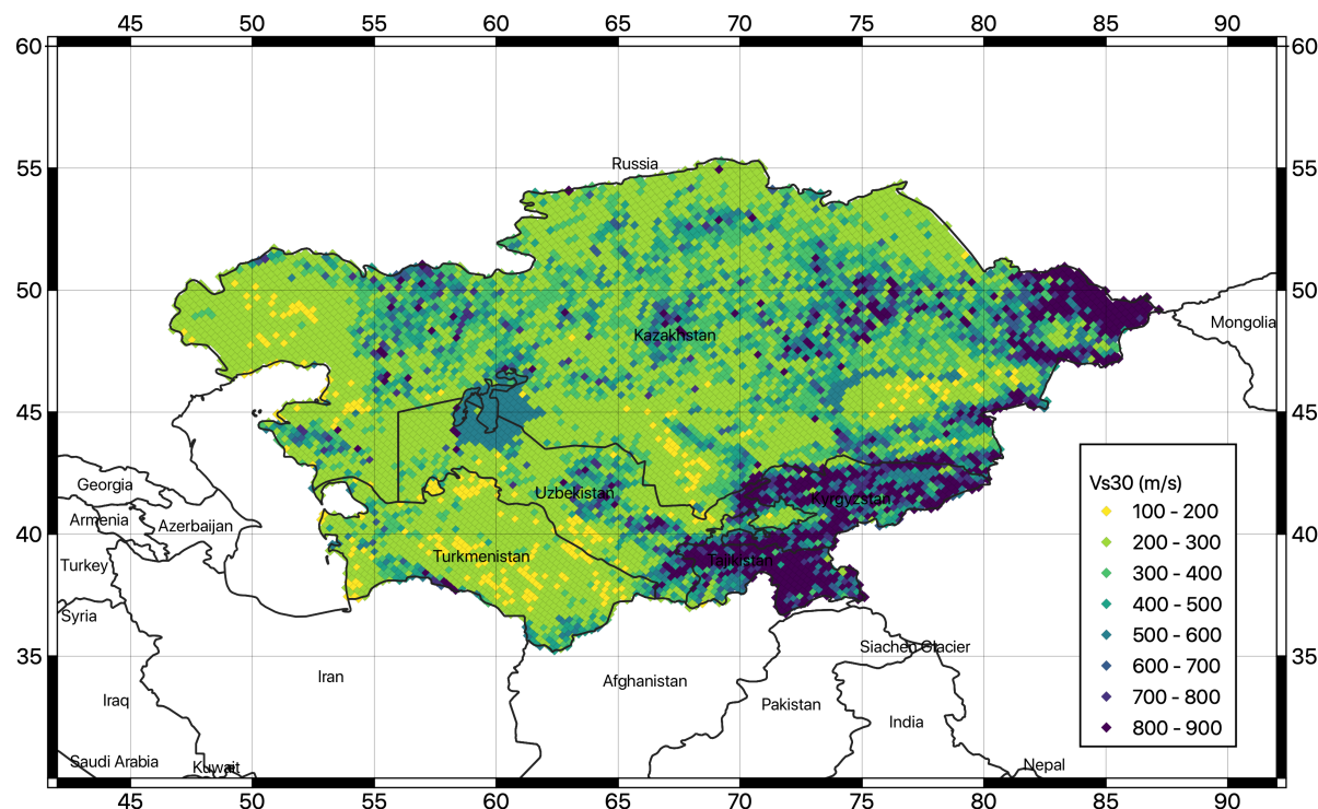
Рисунок 40. Карта значений Vs30, полученная для исследуемой территории
