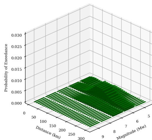
Рисунок 39. Гистограммы дезагрегации для 6 выбранных площадок для спектрального ускорения 0,2с с 10% вероятностью превышения расчетных значений в течение 50 лет (период повторяемости 475 лет)
