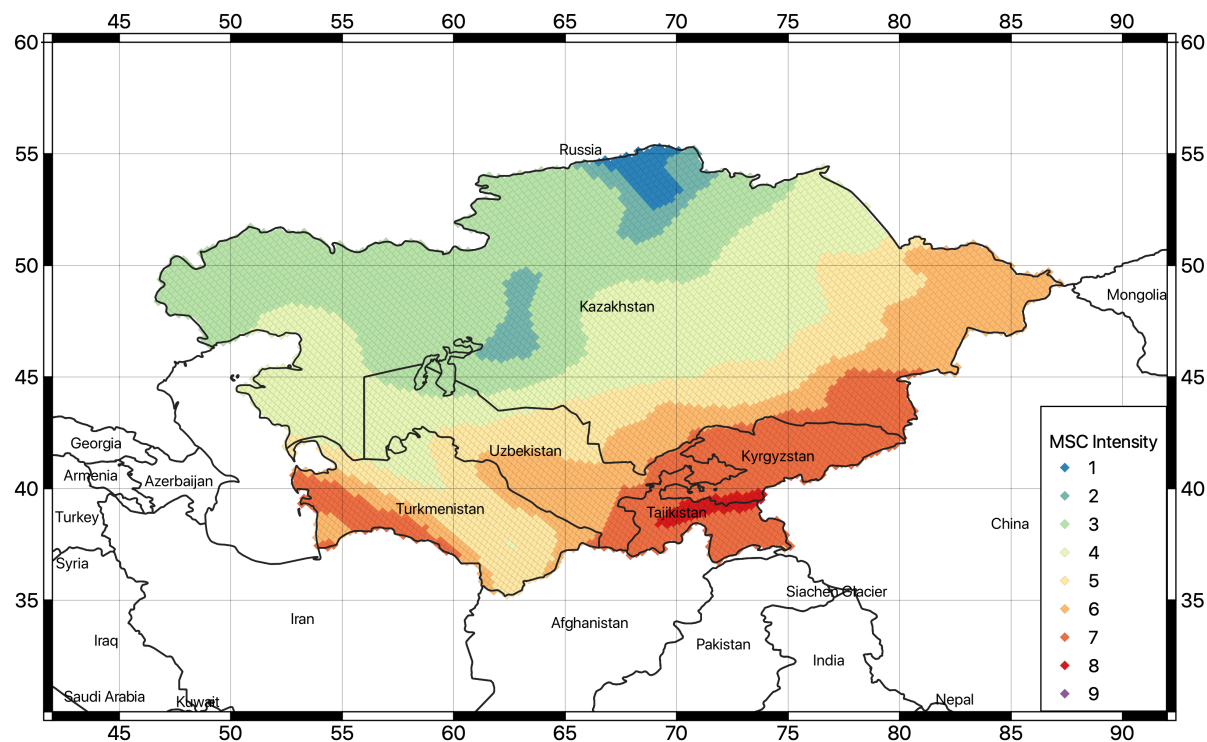
Рисунок 37. Карта в значениях конвертированной макросейсмической интенсивности для 63% вероятности превышения расчетных значений в течение 50 лет (соответствует периоду повторяемости 50 лет)
