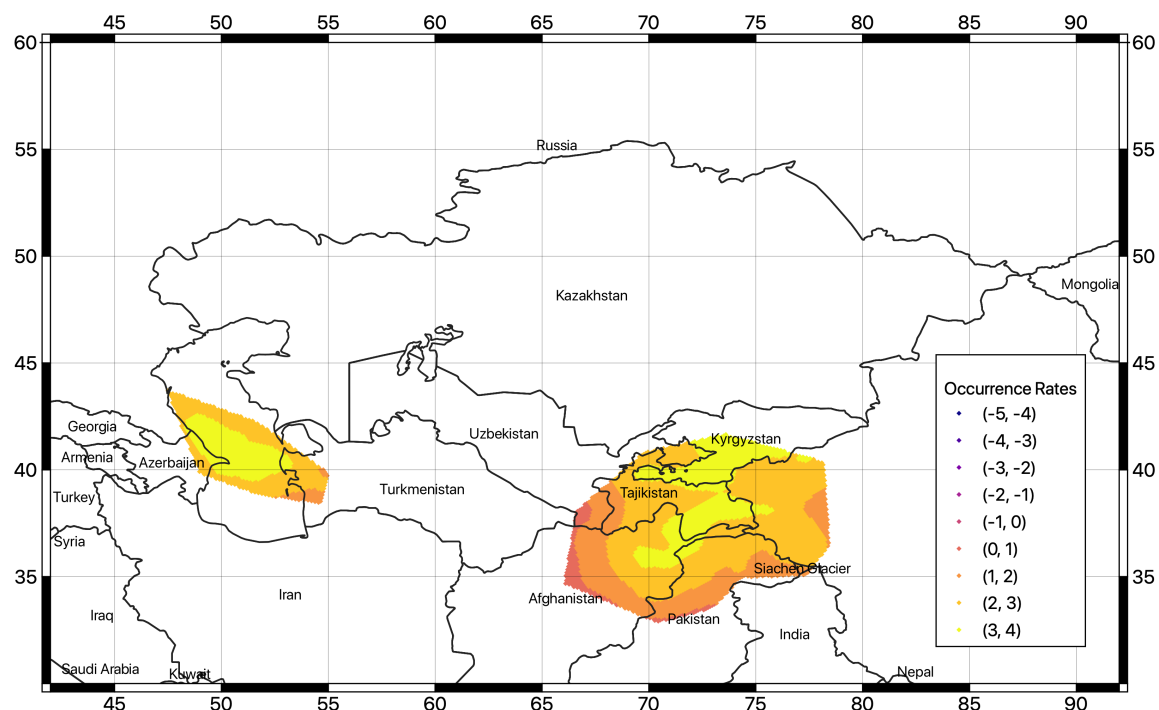
Рисунок 17. Пространственное распределение степени проявления событий в сглаженном виде для зон средне-глубинных землетрясений. Посчитаны с учетом среднего значения весов длины шага сглаживания из Таблицы 13.
