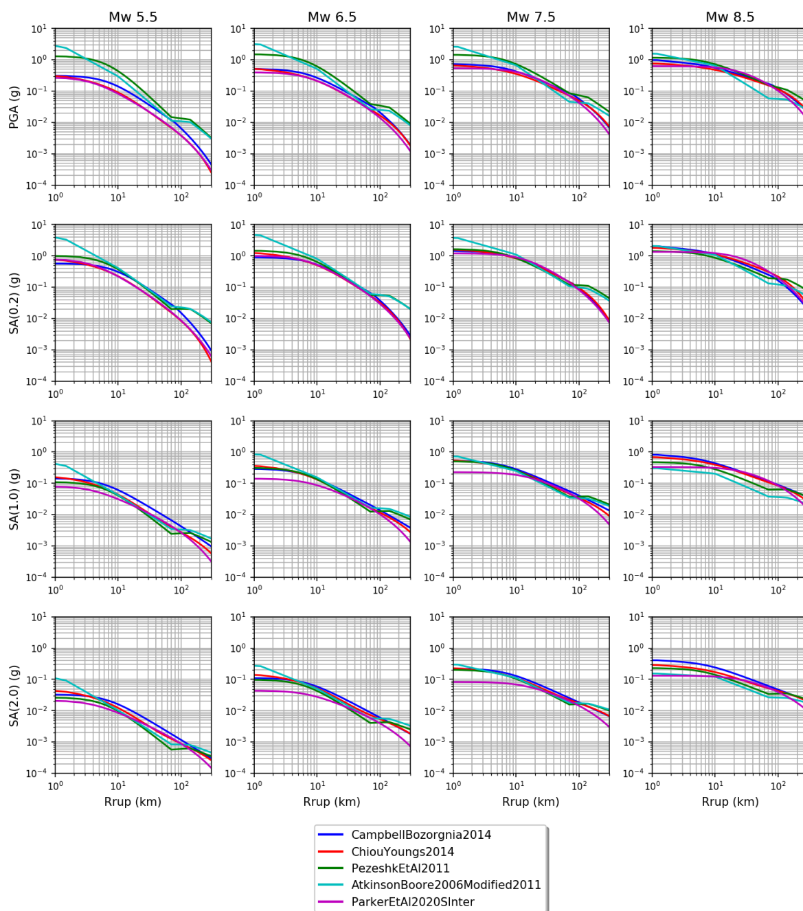
Рисунок 25. Сравнение затуханий движений грунта с расстоянием, даваемых выбранными прогнозными моделями, при различных магнитудах (столбцы) и мерах интенсивности (строки). В моделях для стабильной коры (SC) на расстоянии около 100 км хорошо видно типичное отклонение движений грунта из-за рефракции на границе Мохо
