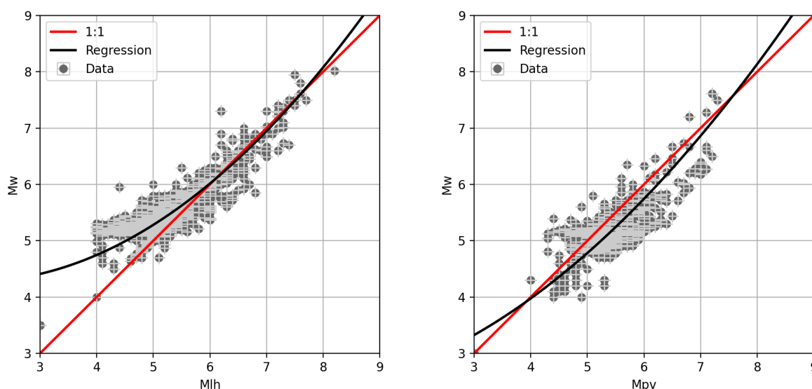
Рисунок 3. Зависимости, разработанные для преобразования магнитуд M_{lh} и M_{pv} в M_w путем подгонки полинома 2-й степени к наблюдаемым магнитудным парам с использованием метода ортогональной регрессии (наименьших квадратов) (таблица 7)
