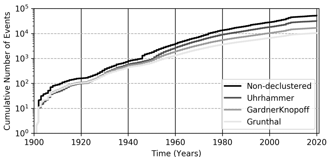
Рисунок 7. Кумулятивное количество событий в зависимости от времени для полного (недекластеризованного) каталога HECCA и для трех каталогов, полученных с помощью трех рассмотренных алгоритмов декластеризации
