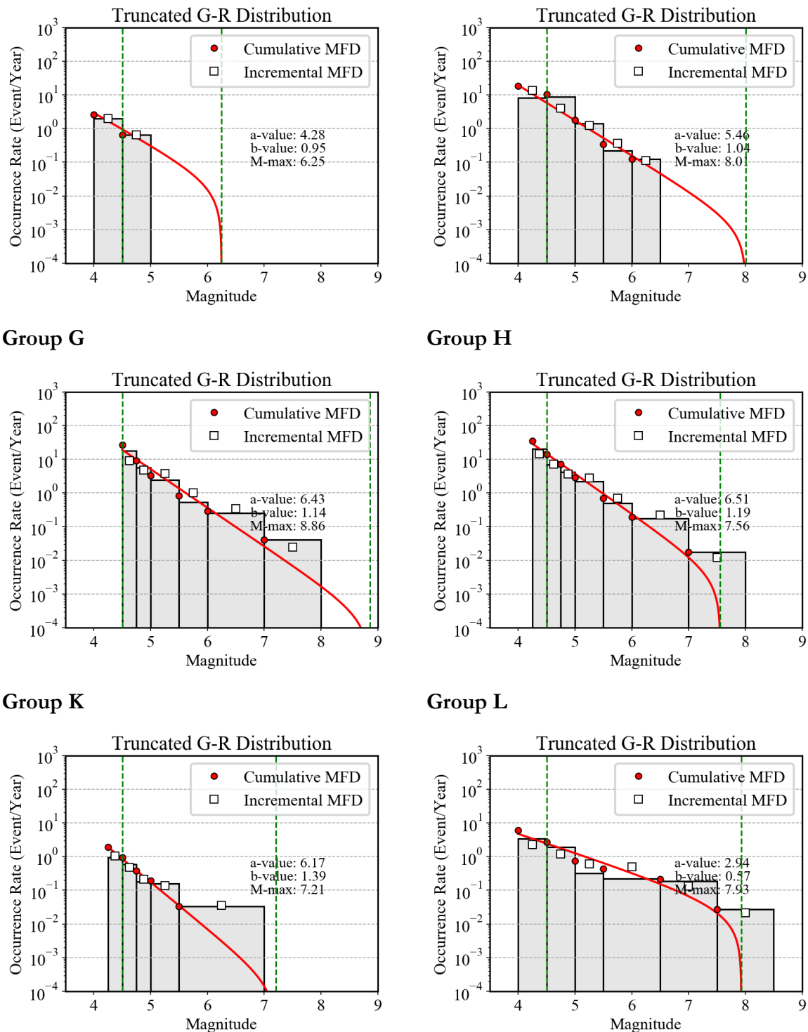
Рисунок 12.. Параметры уравнения Гутенберга-Рихтера, откалиброванные для групп зон для модели Центральной Азии.
